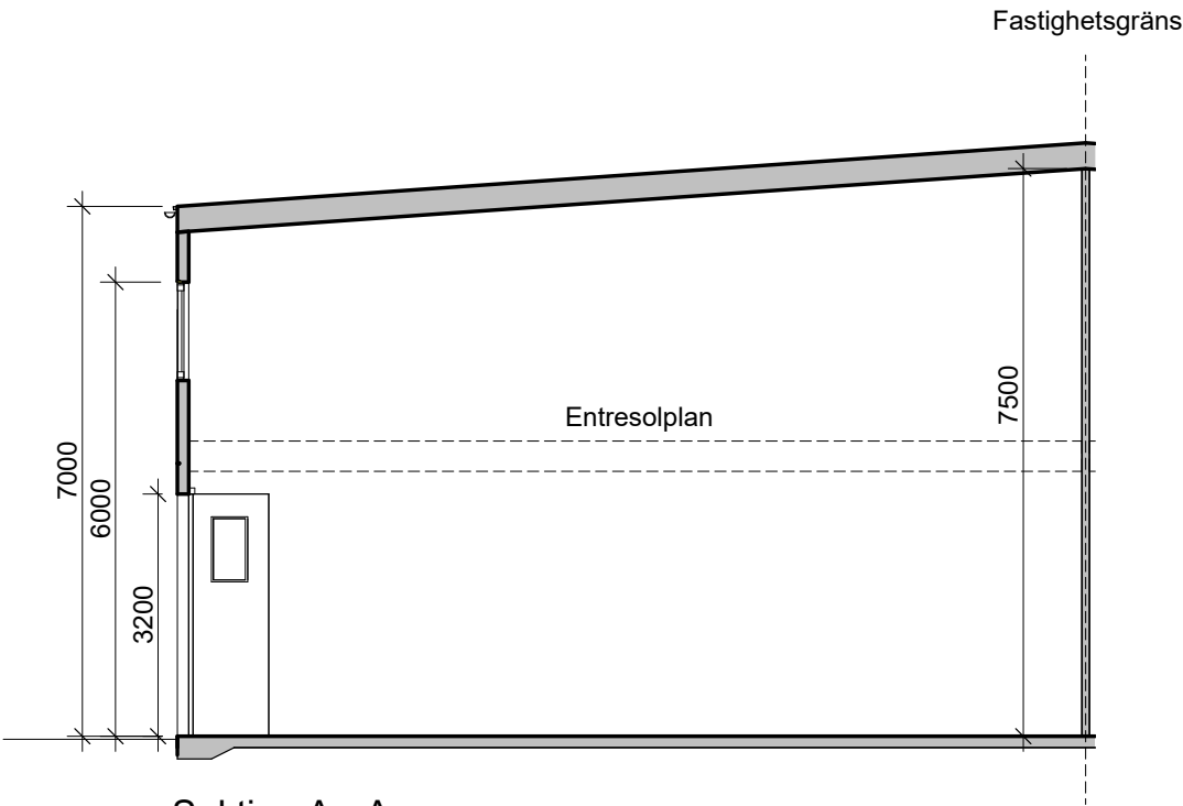
Sektion A - A
