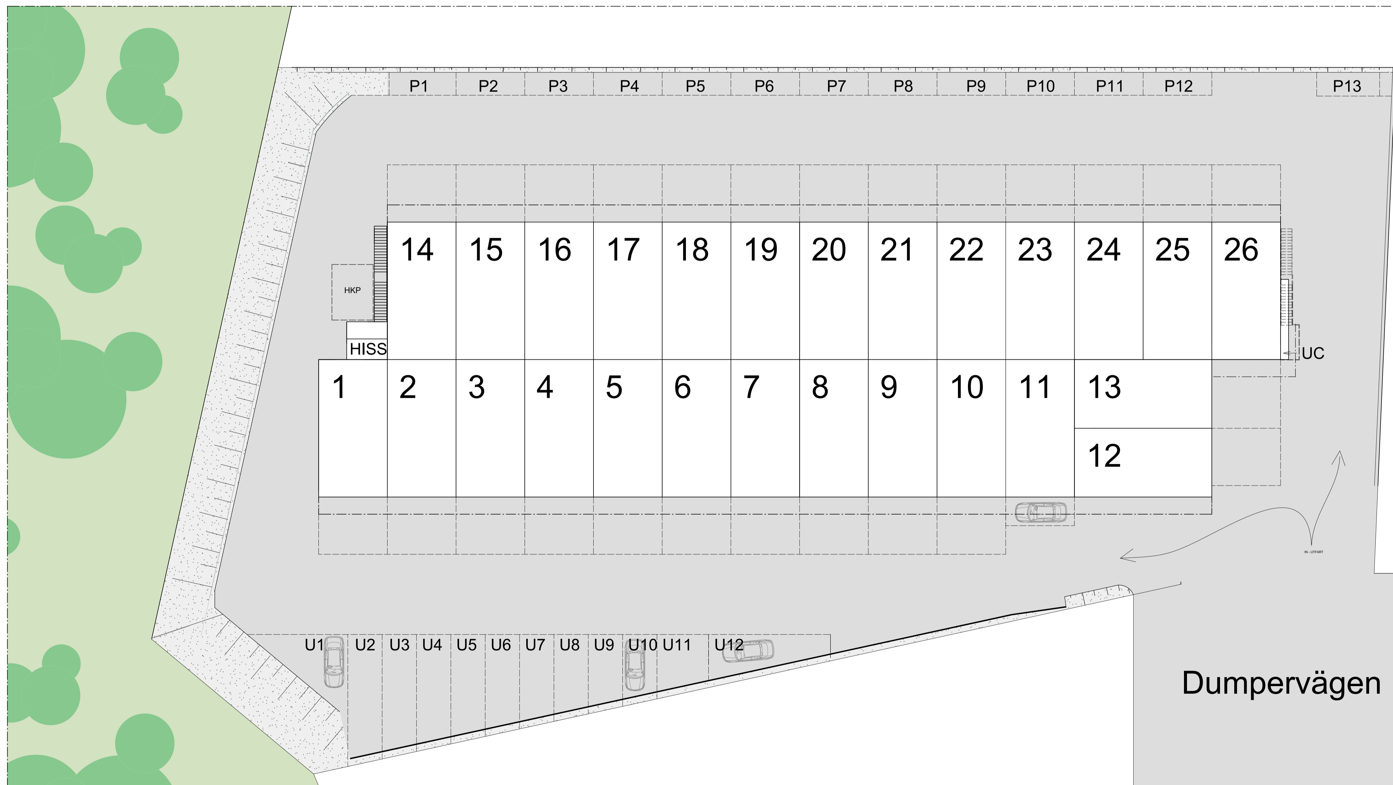
LÄMNA INDUSTRIOMRÅDE SÄJLSITUATIONSPLAN
